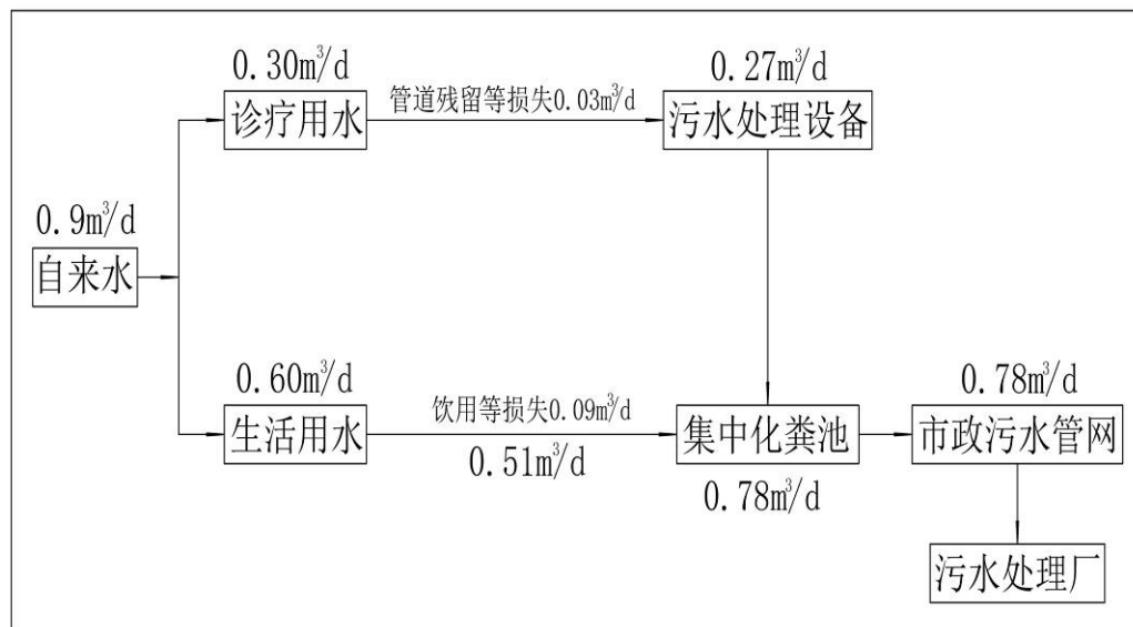
图 3 项目水平衡图
