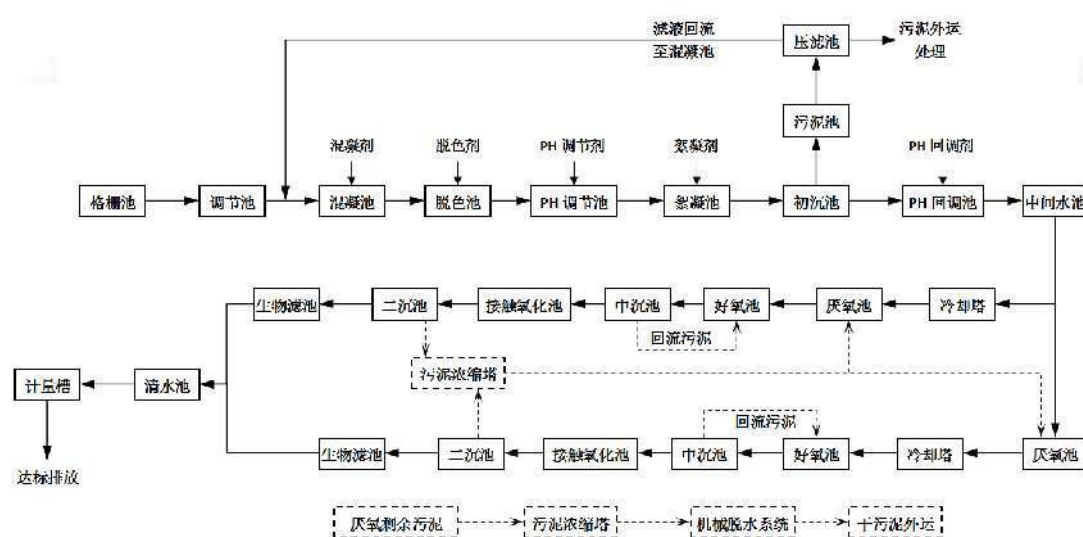
图 2.5.1-1 废水处理工艺流程图
