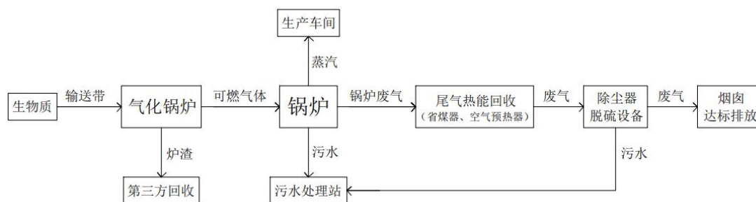
图 2.5.2-1 废气处理工艺流程图
