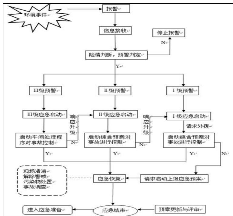
图 6.2.1-1 公司应急响应流程图
