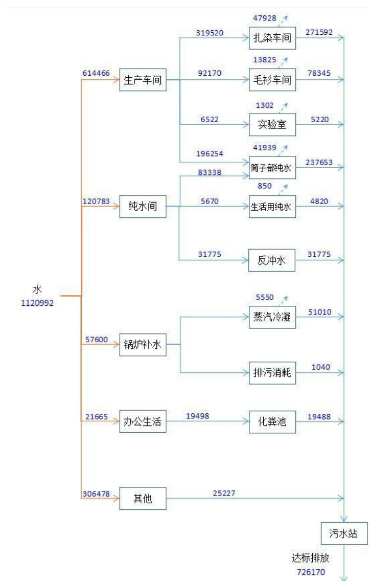
图 2.4.2-1 水平衡图
