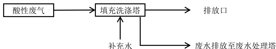
图 3-6 酸雾废气处理工艺流程
