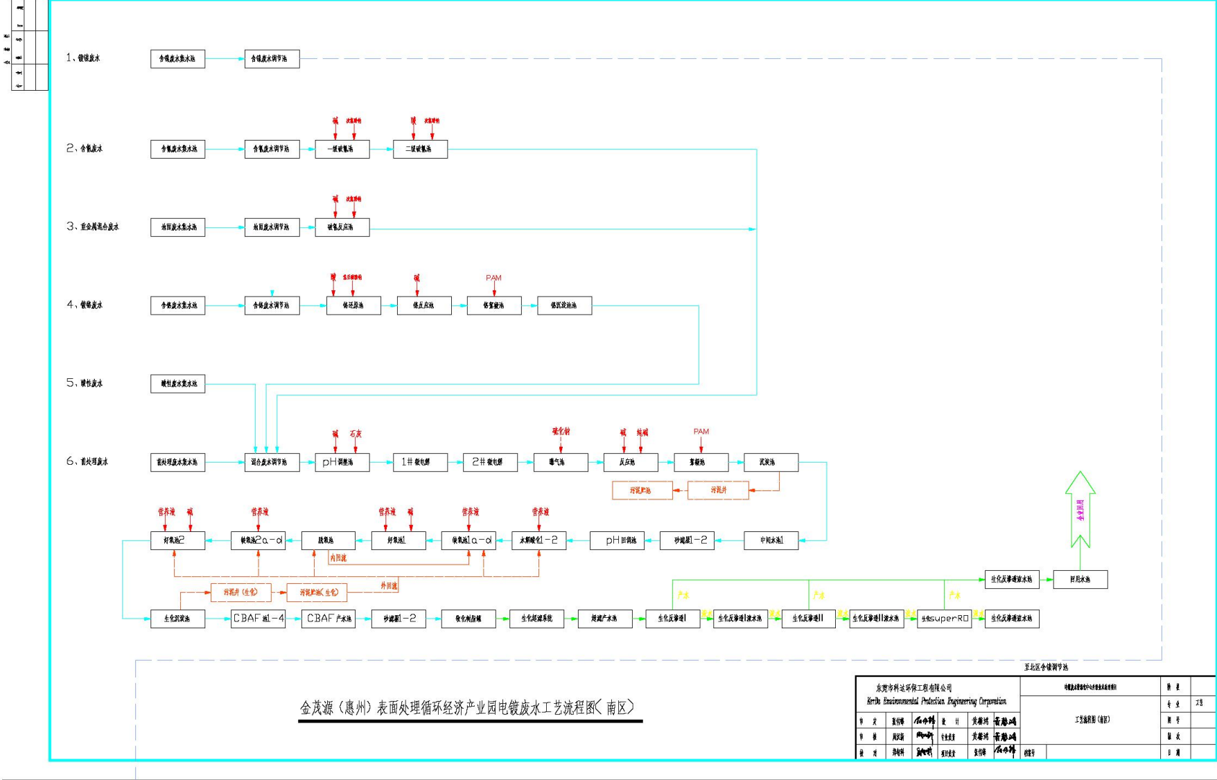
图 3-5 废水处理及中水回用工艺流程图（南区）
