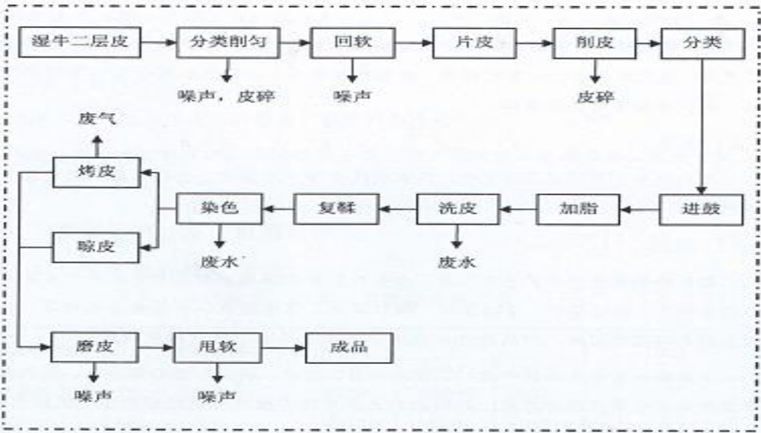
图 2-3 工艺流程图
