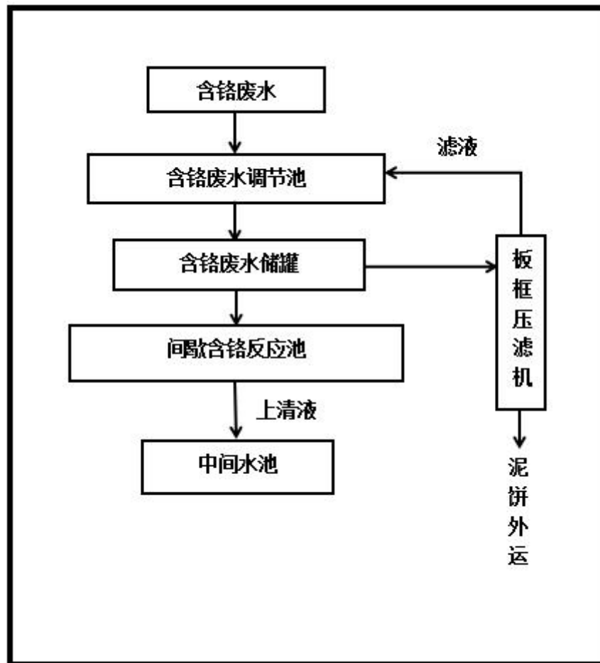
图 2-4 含铬废水预处理工艺
