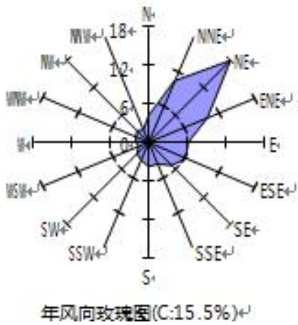
图 2-7 全年风向玫瑰图
