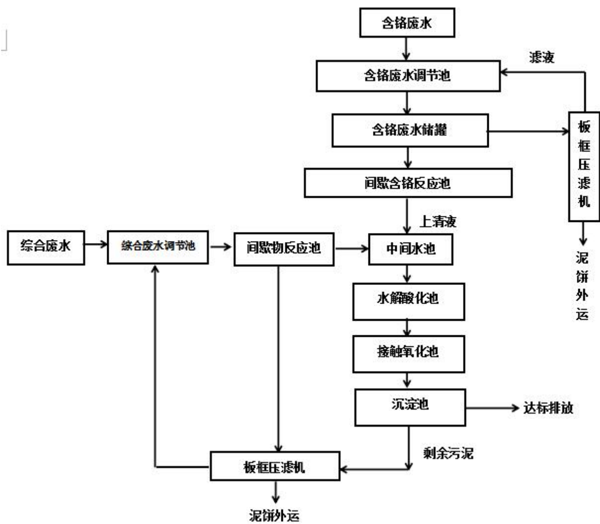
图 2-5 综合污水处理工艺流程
