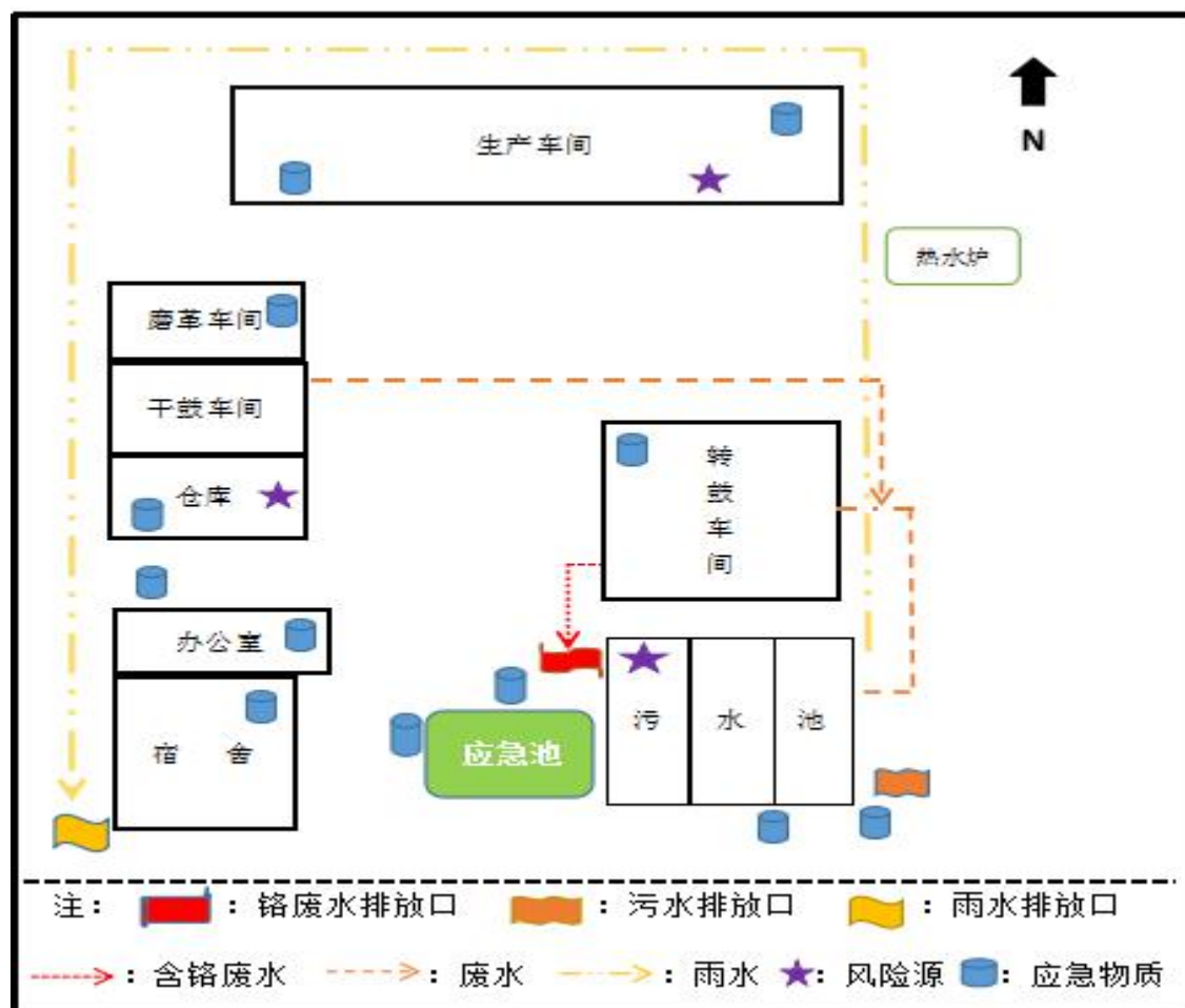
附件 F10：环境风险源分布图
