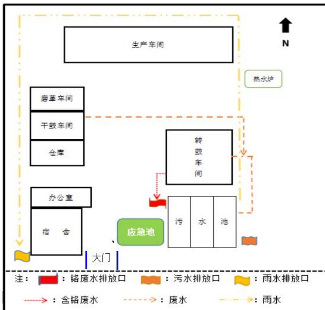
附件 F9：企业雨水、污水管网图
