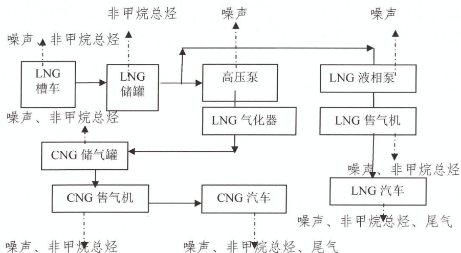
图 3 LNG 加气站工艺流程与产污节点图
